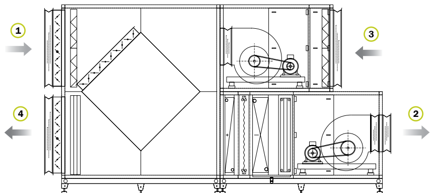
1 наружный (свежий) воздух 2 приточный воздух 3 удаляемый воздух 4 отработанный воздух
