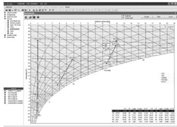
h-x диаграмма
