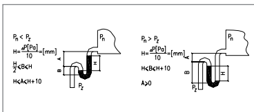
РАСЧЕТ СИФОНОВ СТОКА КОНДЕНСАТА
