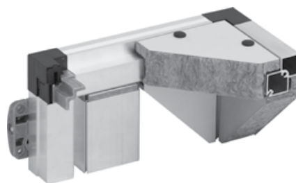
Корпус TopAir
